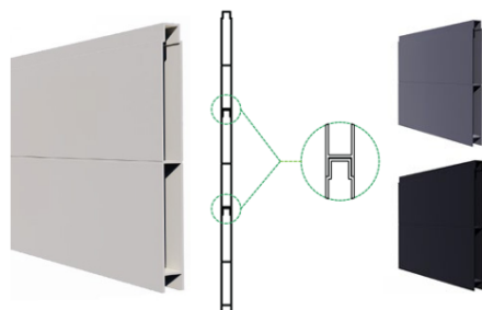
V001018 Panel aluminiowy
