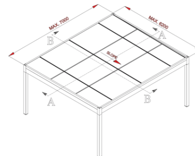
Taras z płaskim dachem Maksymalne wymiary
