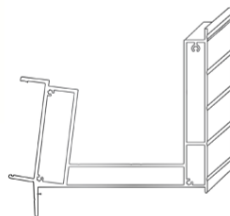
V001001 Nowoczesna rynna z paskami
