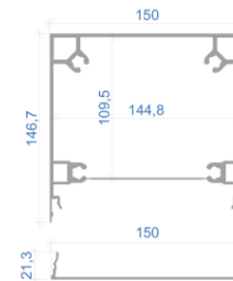
Słupek Wymiary
