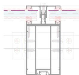
Krokiew Wymiary
